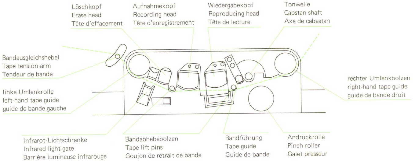
Bandlauf am Kopfträger Tape path across heads Passage de la bande dans le bloc de têtes
